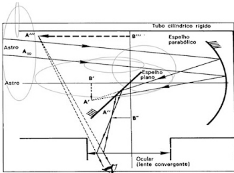
Fig. 4 Esquema para determinação da imagem no telescópio.
