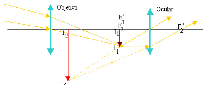
Fig. 3. Esquema para a determinação da imagem formada pela luneta astronômica.
